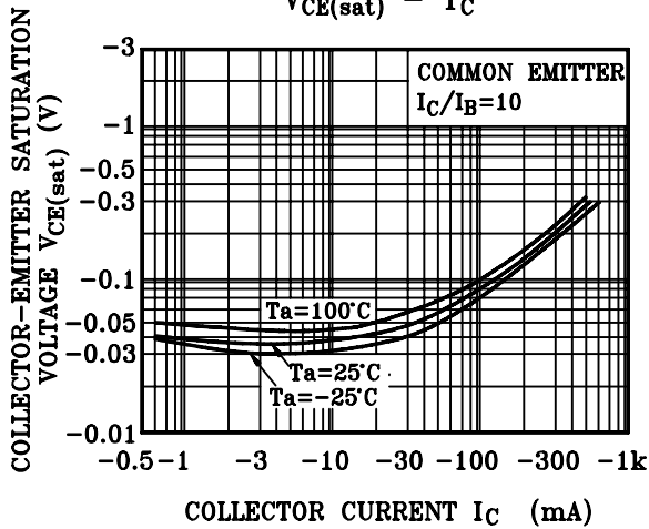
V_{CE(sat)} - I_C
